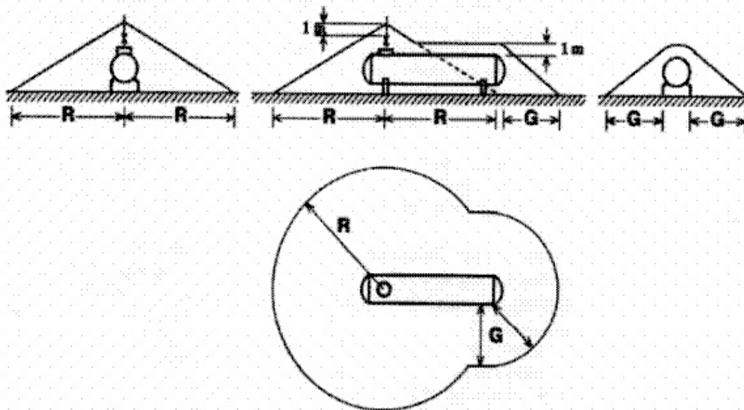
Bild 1: Schutzzone für einen oberirdisch aufgestellten Flüssiggas-Behälter
